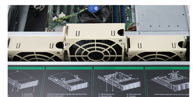
Hot-swap Fan Module
