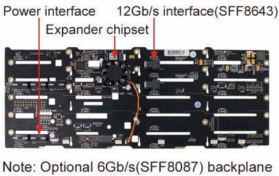
Note: Optional 6Gb/s(SFF8087) backplane
