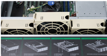
Hot-swap Fan Module
